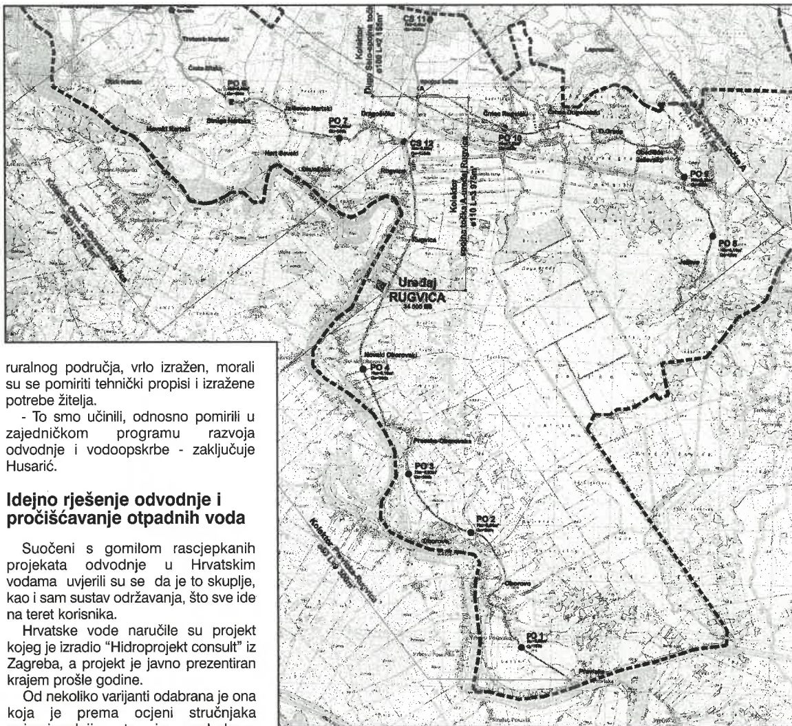
Prikaz optimalnog projekta odvodnje i pročišćavanja otpadnih voda
